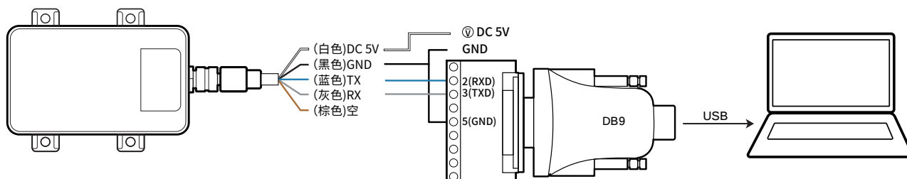
图 6. L4s/L4s-Filled 接 DB9 接线图 (棕色线不接)
