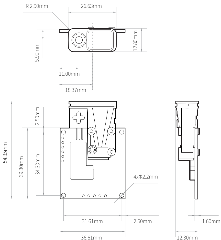
图 8. L4 尺寸图
