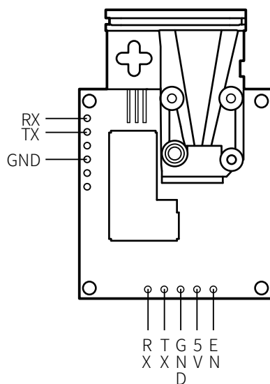
底下 5PIN 2.54mm 单列针 / 孔接口
