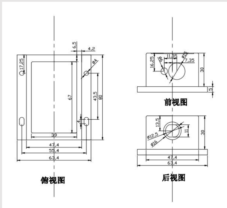
SLDS-A30PW 激光测距传感器
