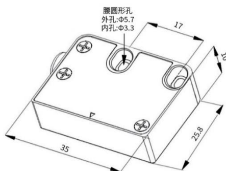
图 1-1: 产品尺寸 (单位: mm)
