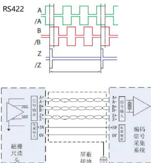
图 1-2: 输出信号
