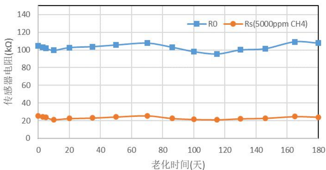
图4 传感器的长期稳定性曲线
