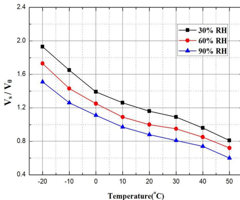
图3 传感器的温度，湿度特性曲线
