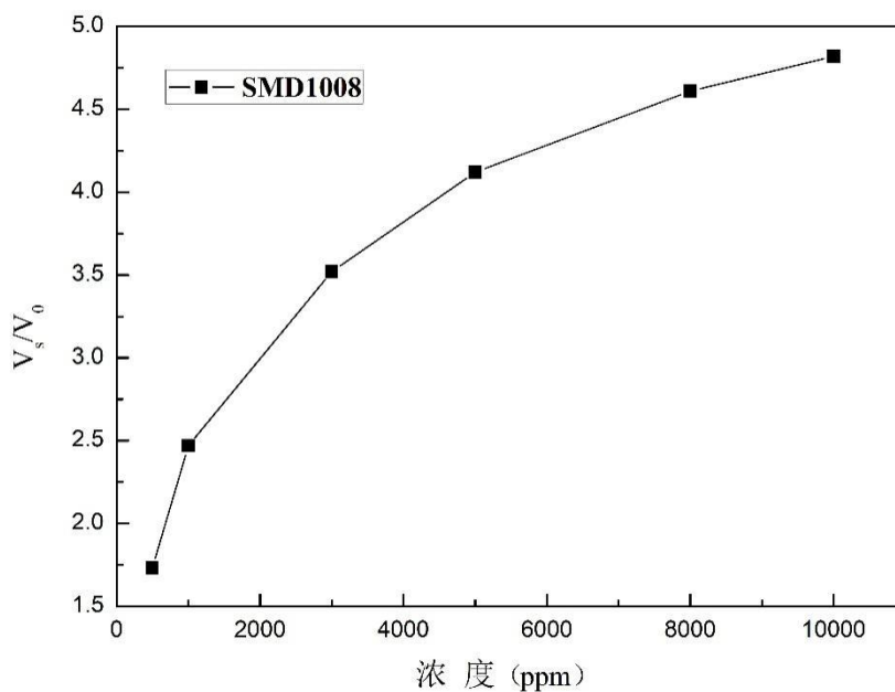
图 1 甲烷传感器灵敏度特性曲线
