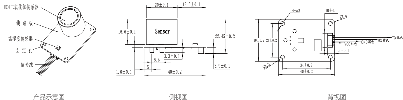
TB200B-EC4-CIO 2 -5-01尺寸示意图
