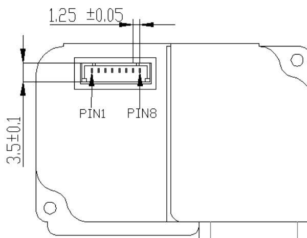
图 2 数字接口管脚定义
