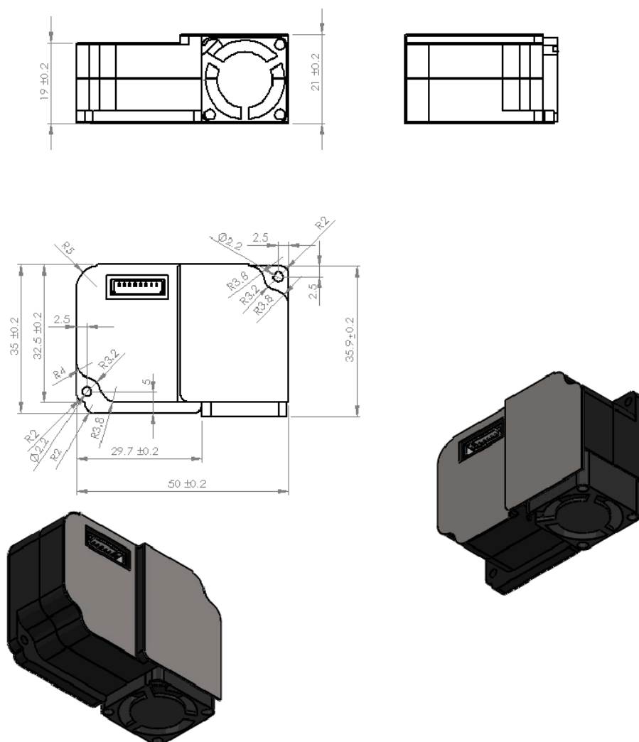
图 4: 外形尺寸 (单位: mm)
