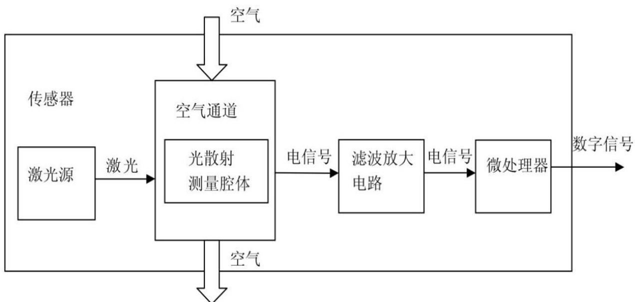
图 1 MMD201A 传感器功能框架图
