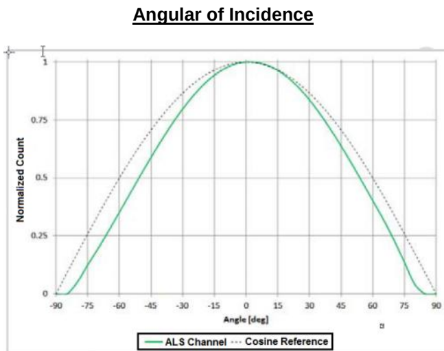
Figure 4.3 ALS Sensitivity vs. Angular of Incidence
