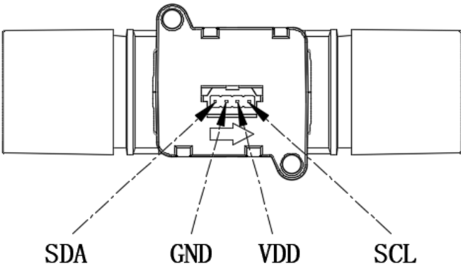
图 2：传感器引脚分布图
