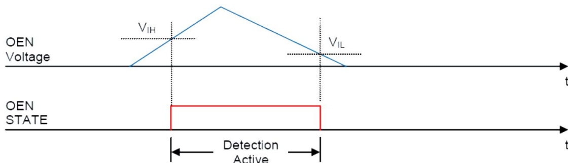
OEM脚滞回电平图
