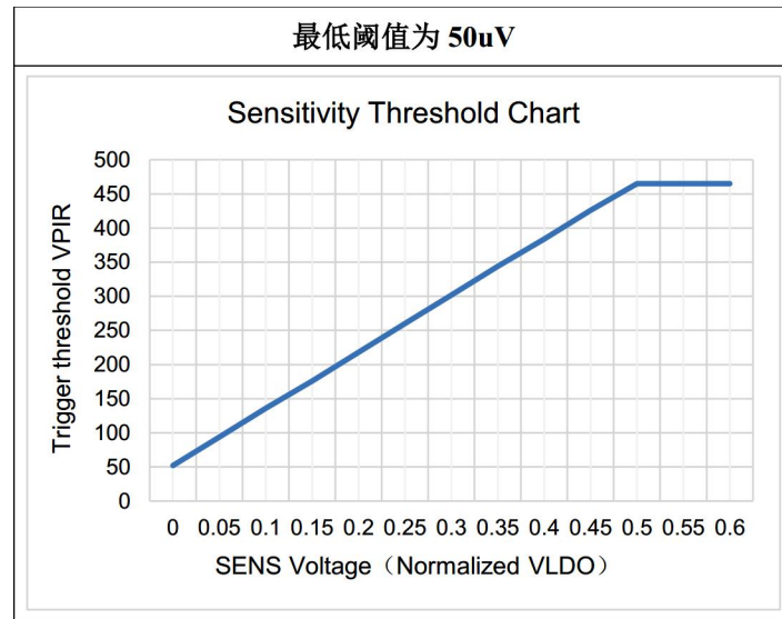
触发阈值与 SENS 电压关系图
