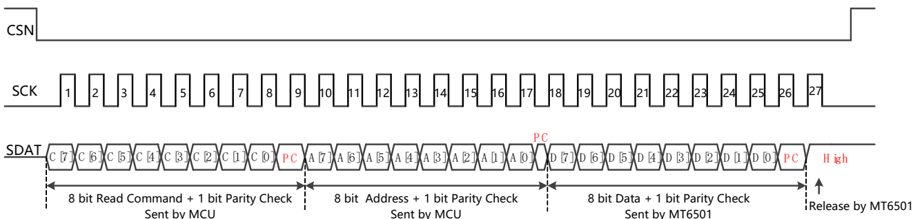
图-12: 3线SPI读取数据时序
