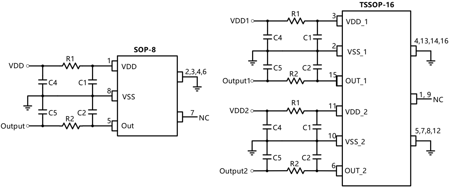
图-14: 模拟输出参考电路 (请确保芯片供电能满足 IDD_{PU} 单路60mA、双路120mA的峰值要求)
