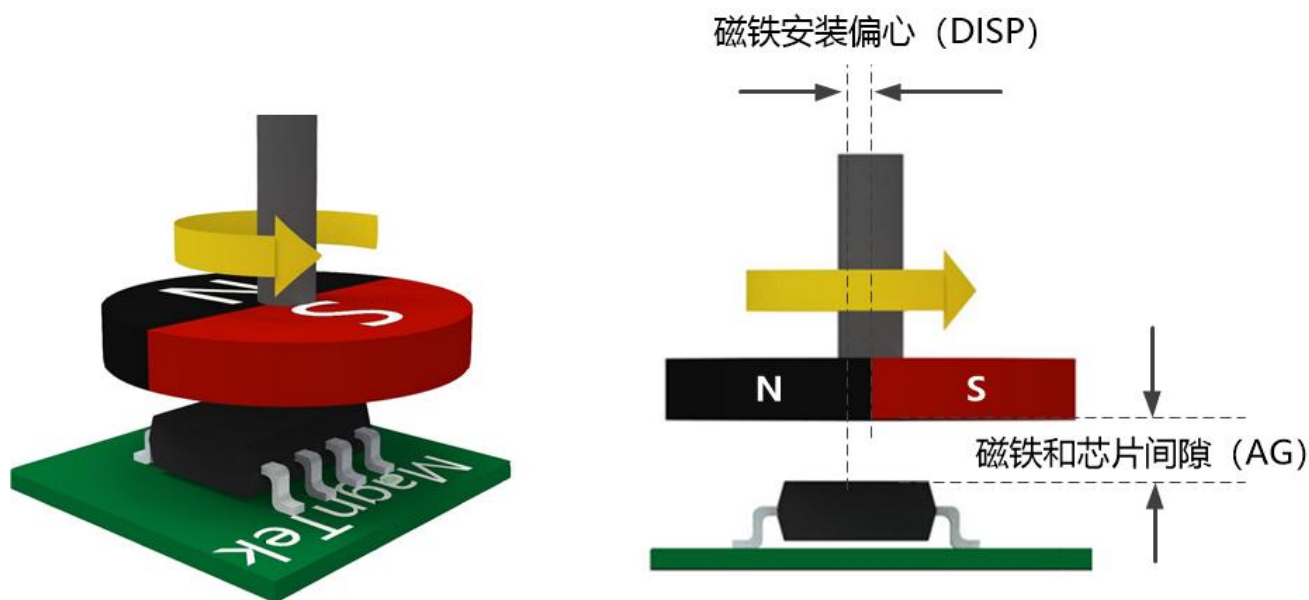
图-5: 磁铁的安装
