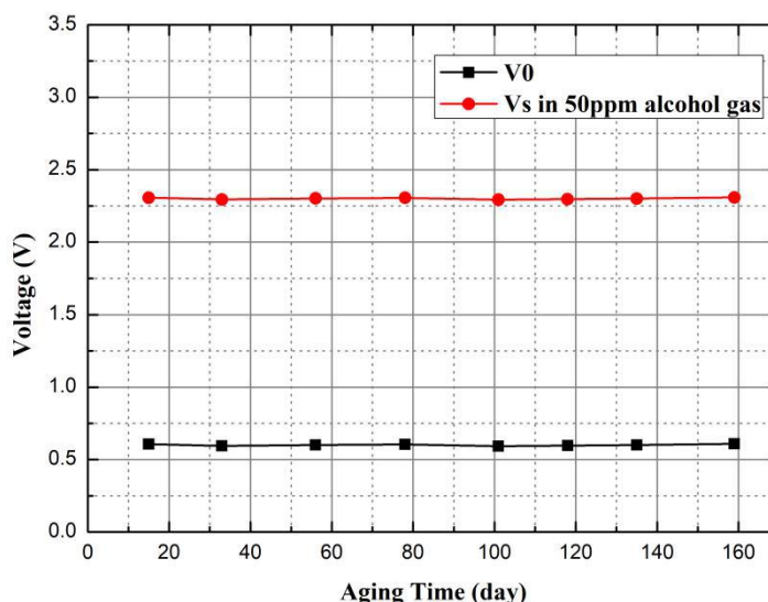
图 3 传感器稳定性曲线
