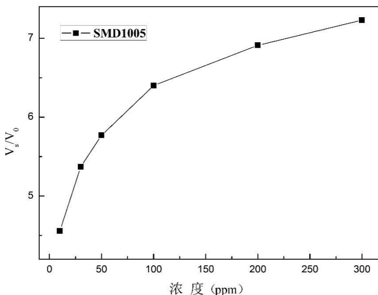
图1 传感器的灵敏度特性曲线
