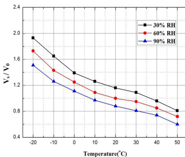
图2 传感器温度、湿度特性曲线
