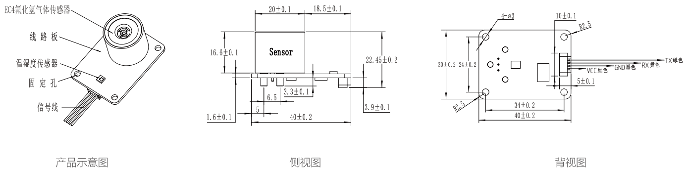
TB200B-EC4-HF-10-01尺寸示意图
