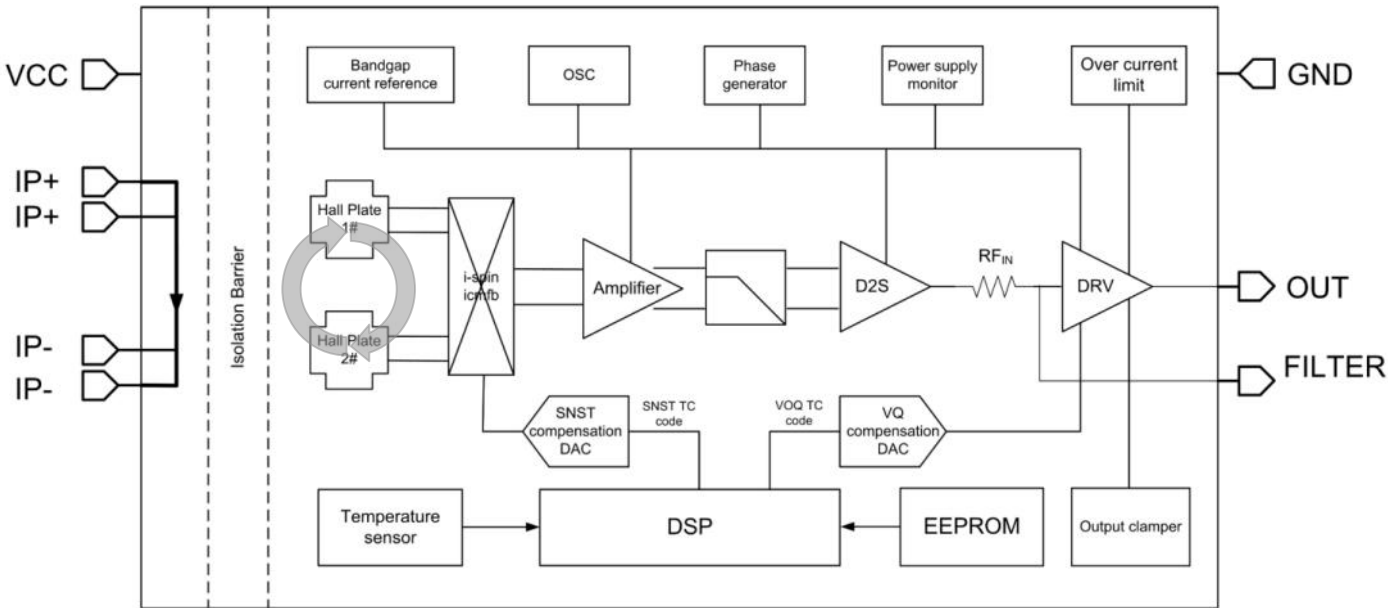
图.1 功能框图
