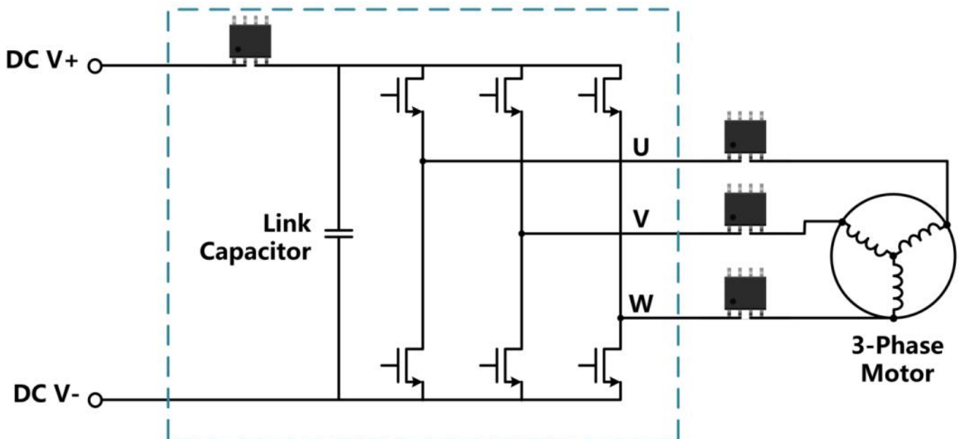
简化三相逆变器原理图
