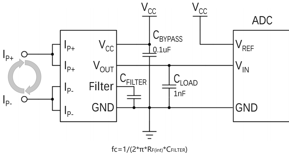
典型应用电路
