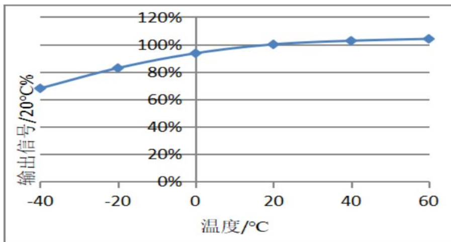
图2: 温补补偿曲线
