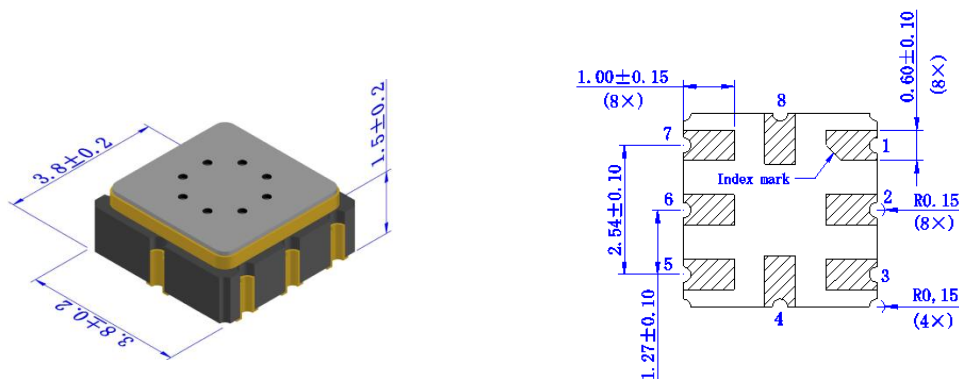
底视尺寸图(单位: mm)
