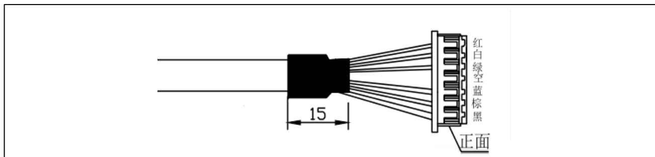
图 2 TF03-100 新版本尾线端子图示
