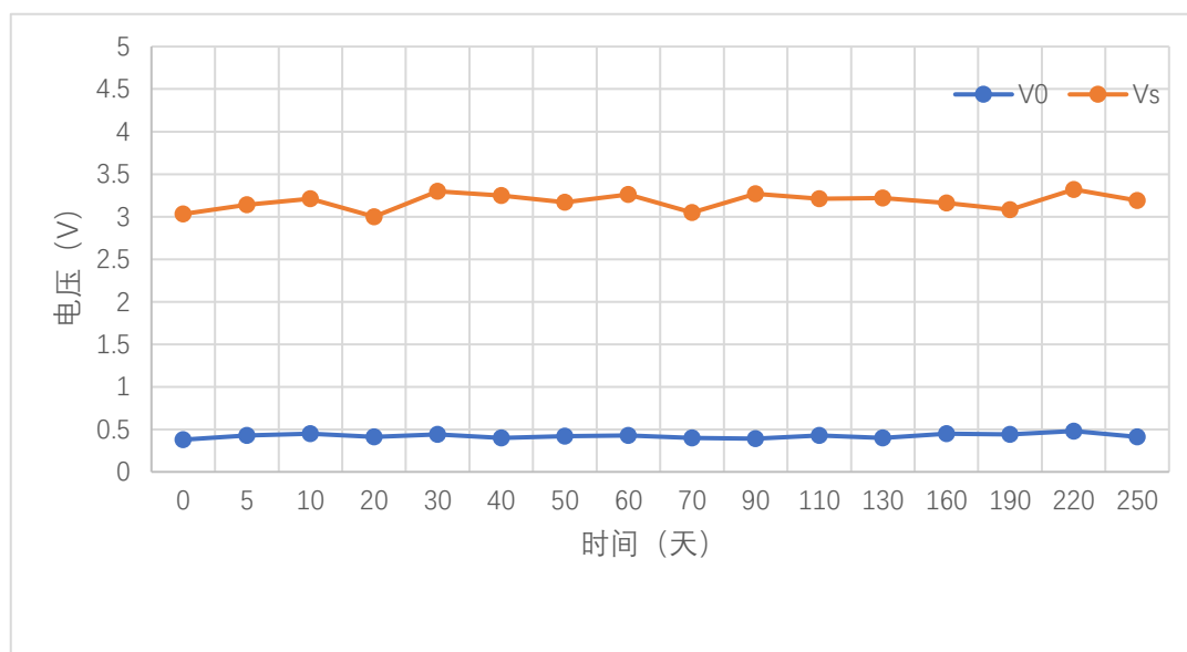
图4 传感器长期稳定性曲线
