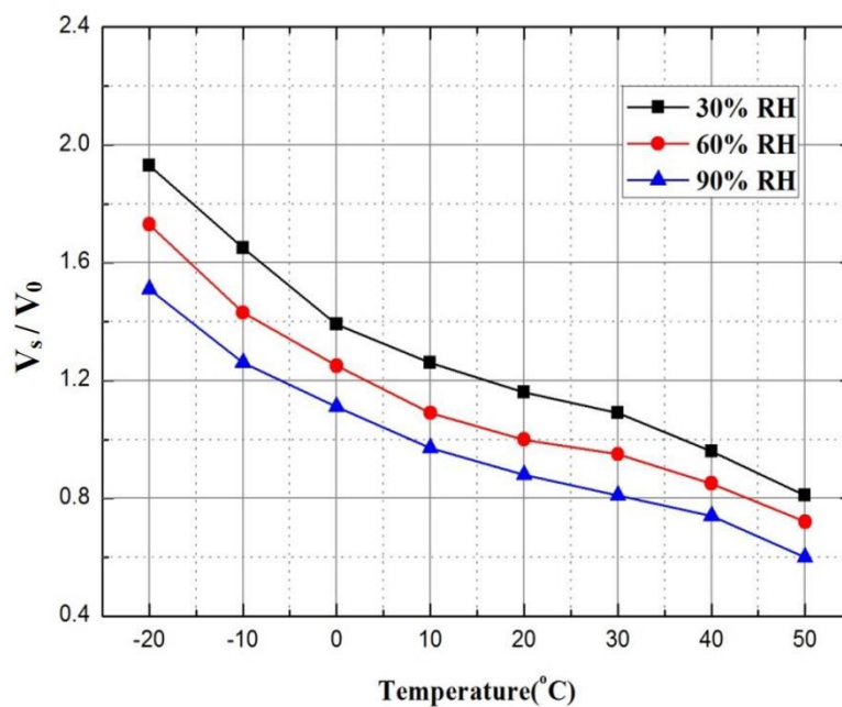
图3 传感器温度、湿度特性曲线
