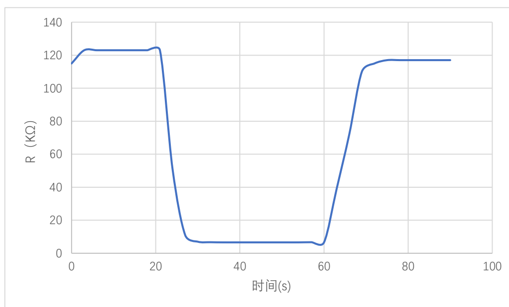
图 2 传感器响应-恢复特性曲线
