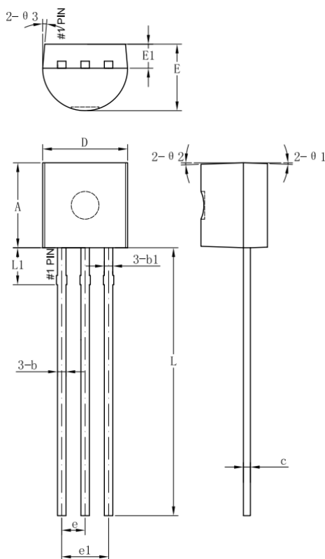
T0-92 外形图
