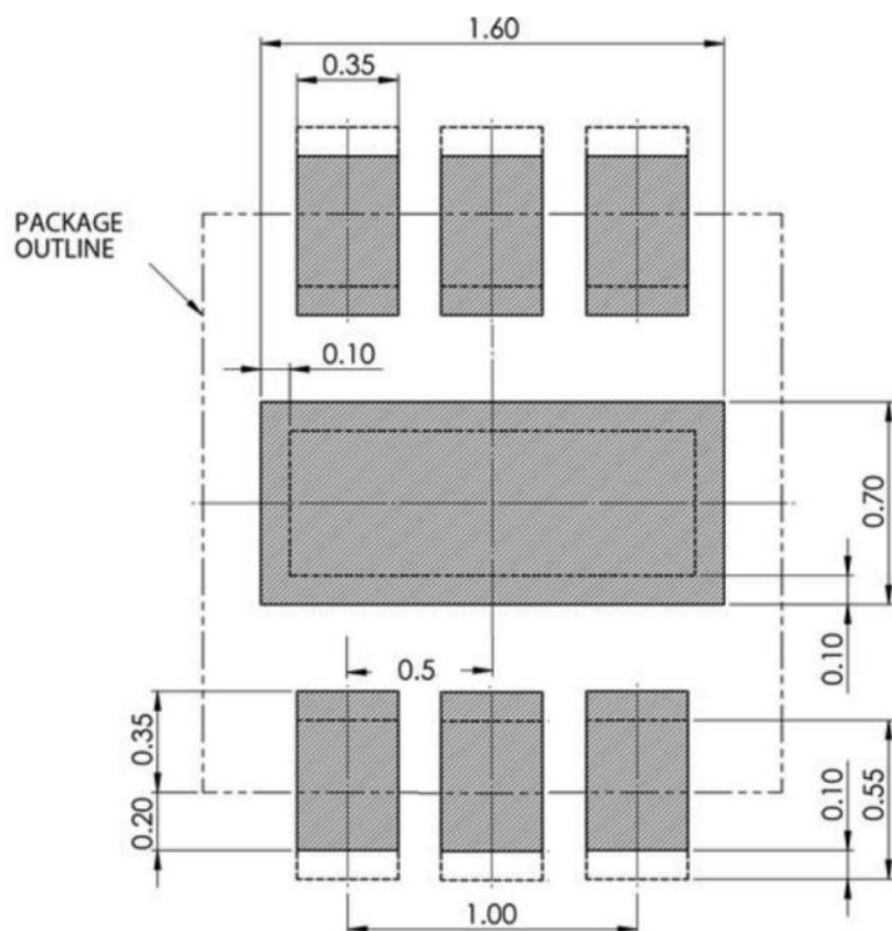
图10 Metal Land Pattern
