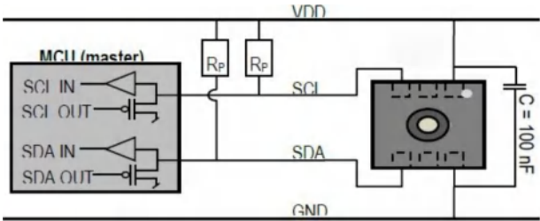
图 6 SHTC3 的典型应用电路，包括上拉电阻和去耦电容 为了机械应力考虑，中心焊盘必须被焊接到地。
