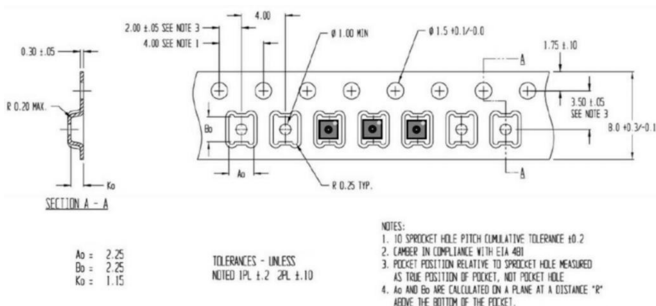
图 11 卷带式封装尺寸
