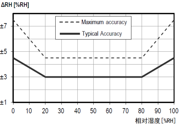
图 2 典型湿度误差和最大湿度误差 (@25℃)
