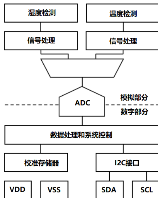
图 1 SHTC3 功能模块示意图
