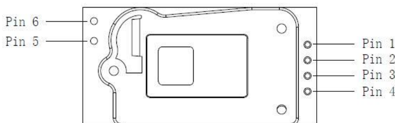
图 3.ACD10 引脚图
