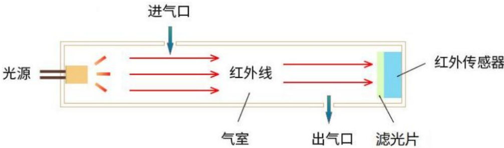
图 2.ACD10 工作原理图
