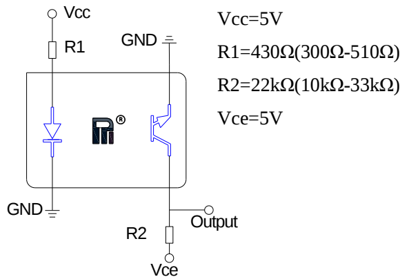
电气原理图
