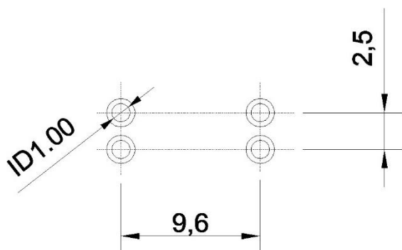
PCB Layout参考图
