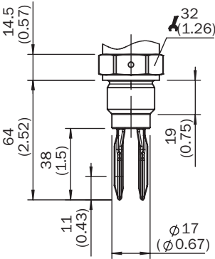
外壳尺寸图
