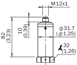
外壳尺寸图
