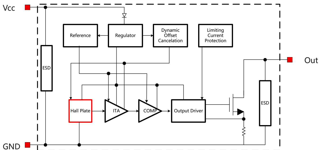
图.5 功能框图
