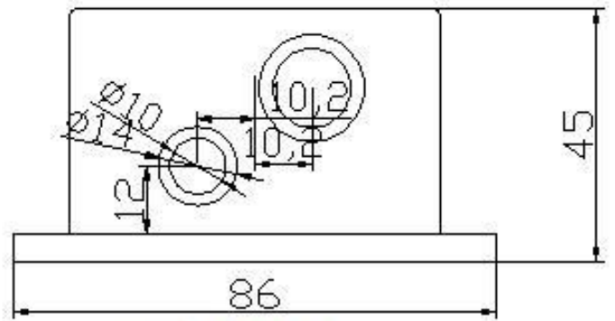
前视图
