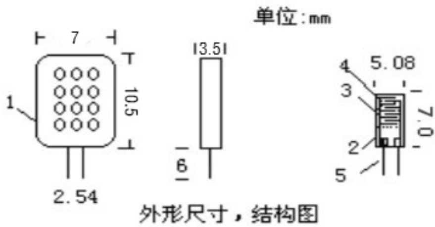
2、小尺寸 S（方形） 图二（单位：mm）
