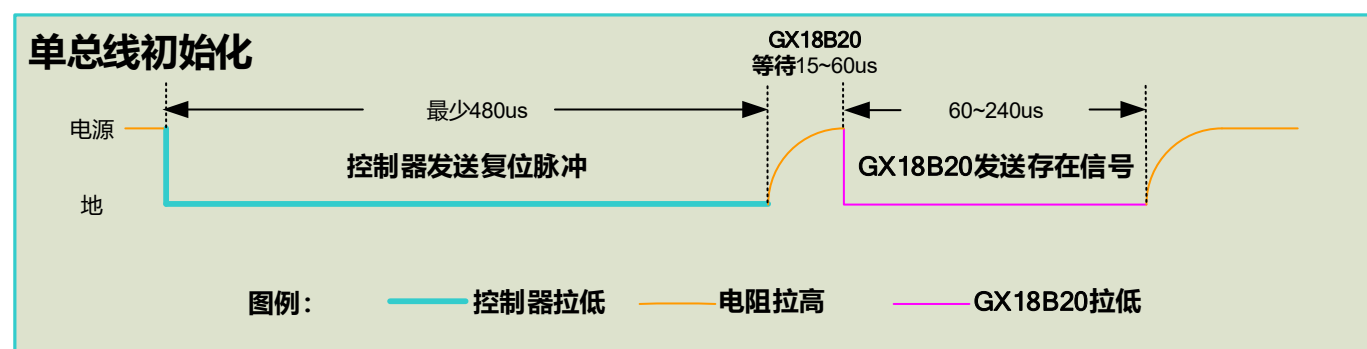
图 13. 初始化序列
