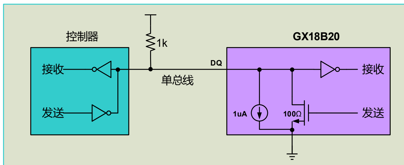
图 10. 硬件结构图
