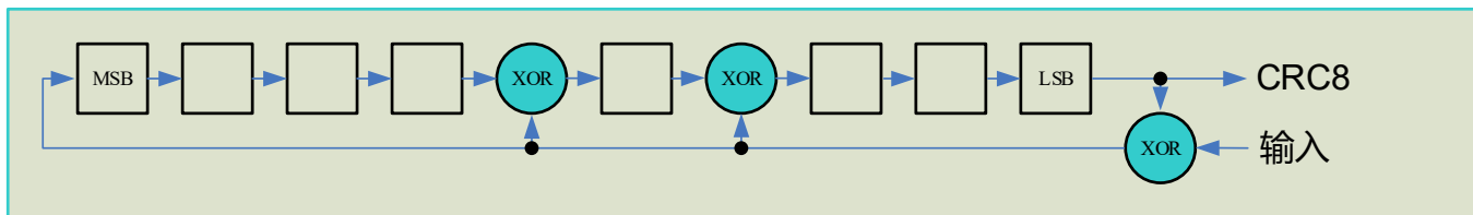
图 9. CRC 产生器
