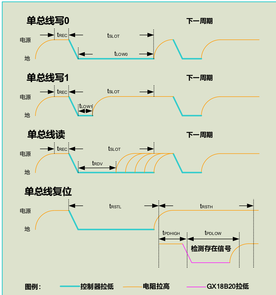
图 18. 时序
