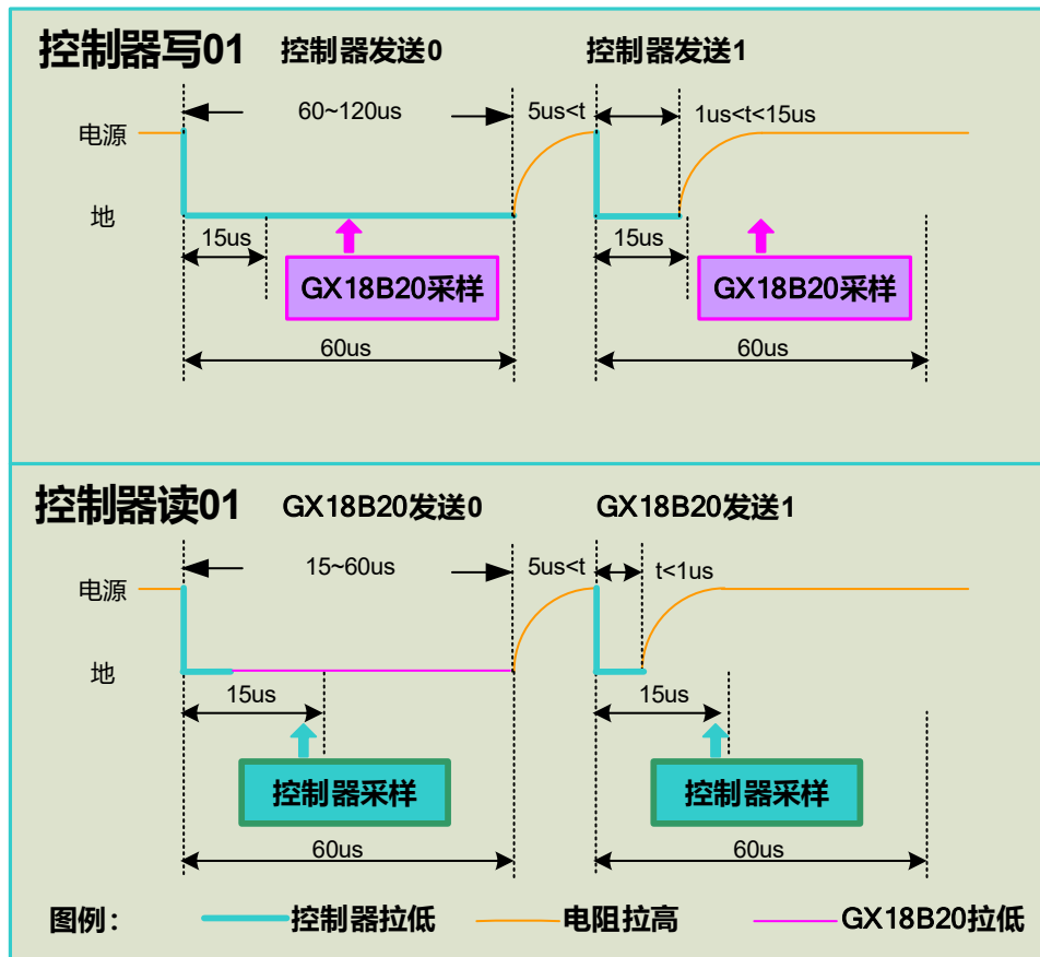
图 14. 读/写时序图
