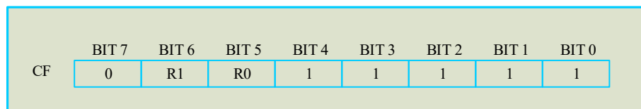
图 8. 配置寄存器
