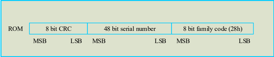
图 6. 64 位 ROM 码
