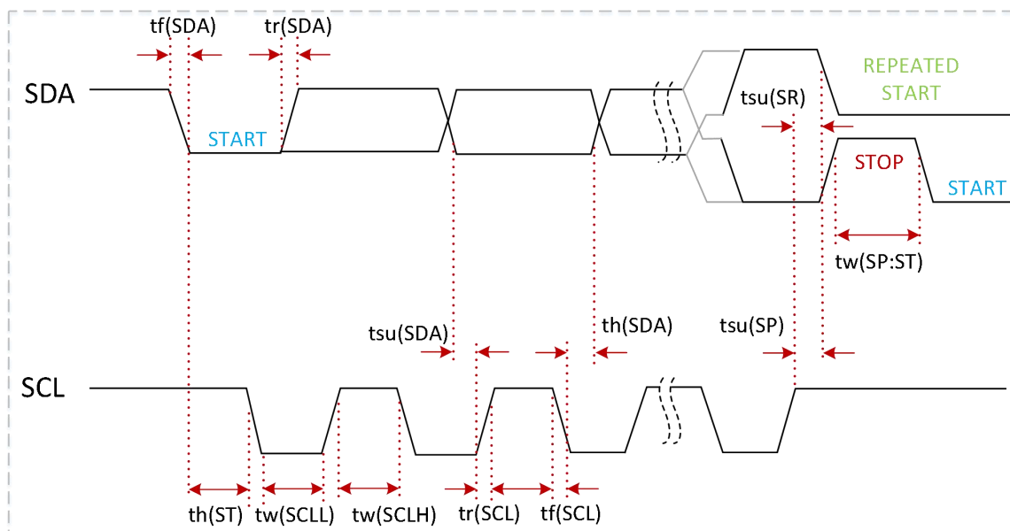
图 13-1 I2C 时序图
