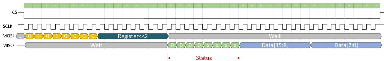
图 15-1. 读寄存器 SPI 时序图
