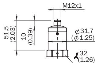
外壳尺寸图
