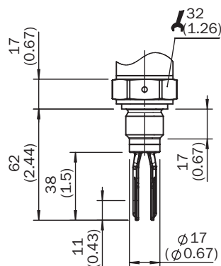
外壳尺寸图
