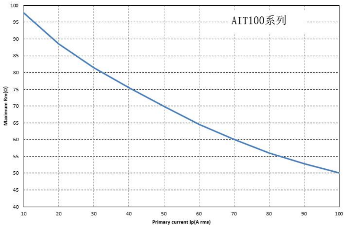
图 1：负载电阻与测量电流关系图
