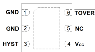
管脚说明
