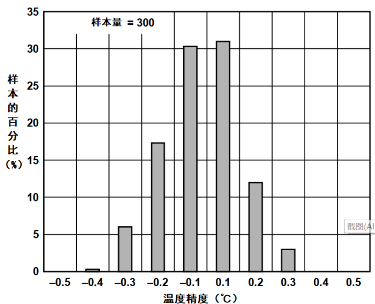
图2 触发阈值精度
