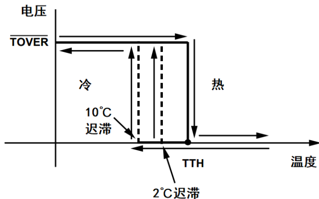
图 6 \overline{TOVER} 功能图解
