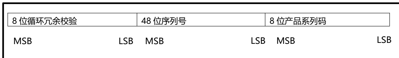
图 9.1 64 位 ROM 编码
