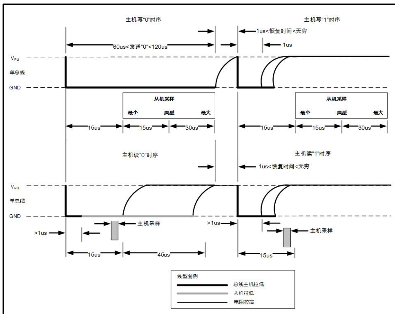
图 10.6-2 读/写时序
