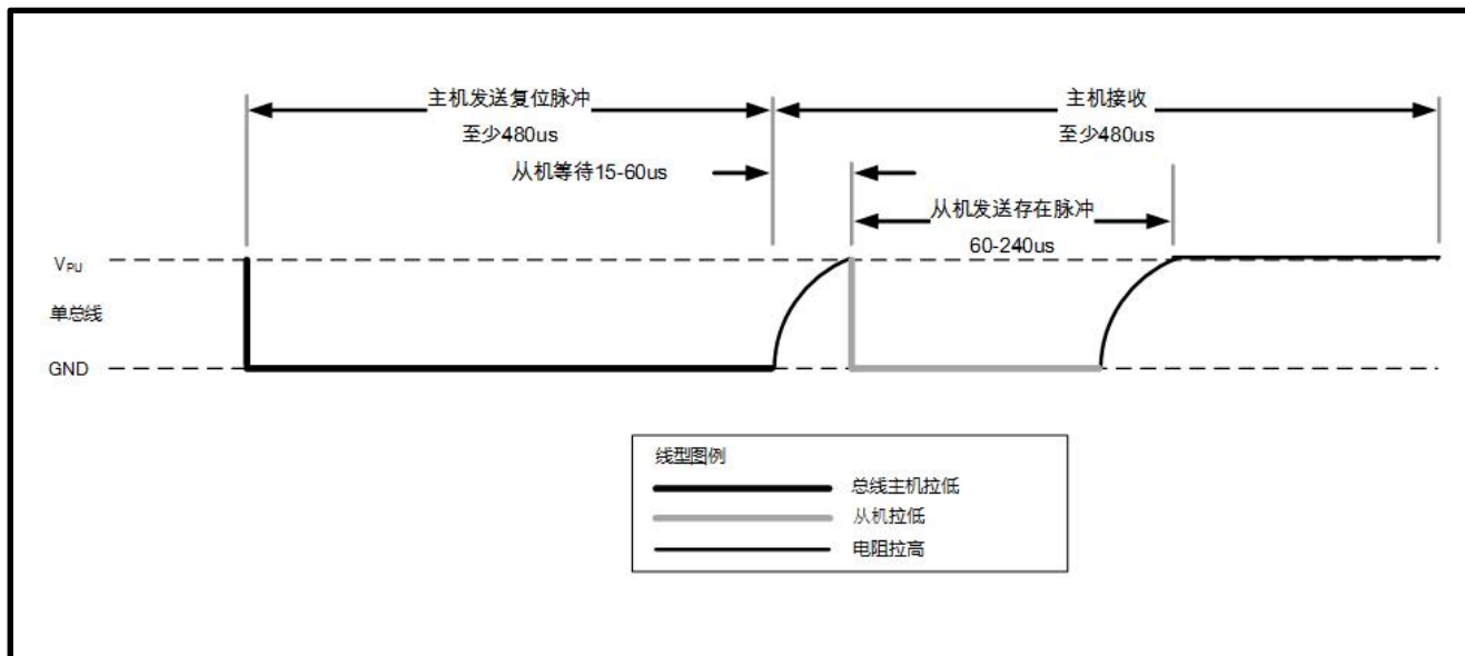
图 10.6-1 初始化时序
