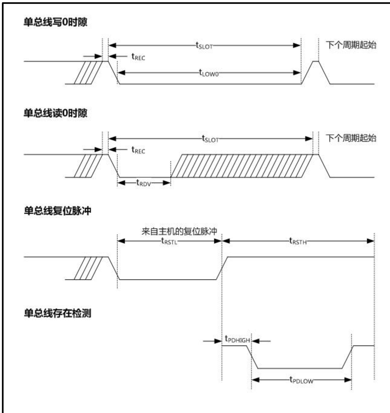
图 10.6-5 时序图
