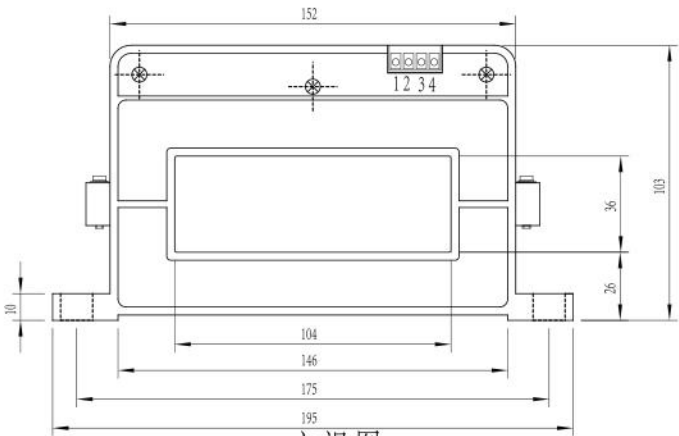
主视图
