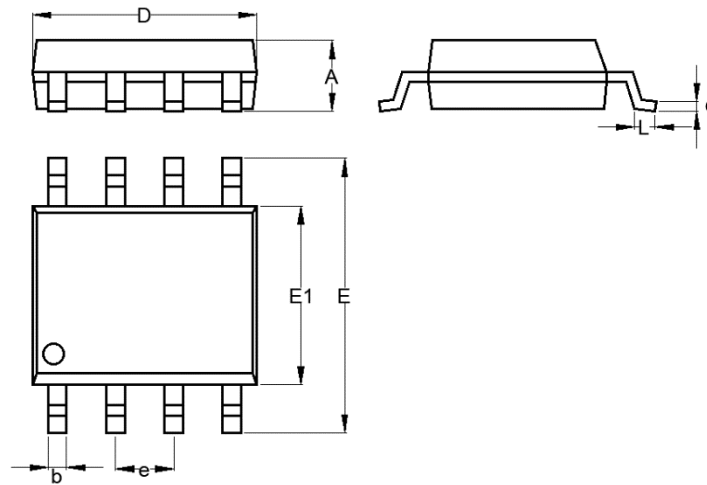
SOP8 外形图
