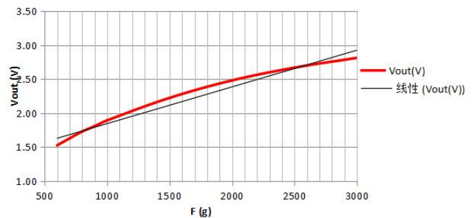
Vout(V)
