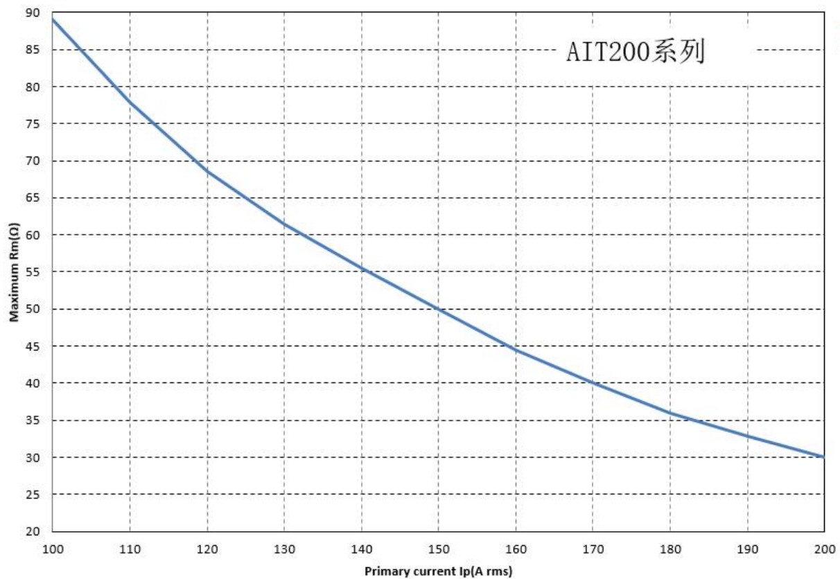
图 1：负载电阻与测量电流关系图
