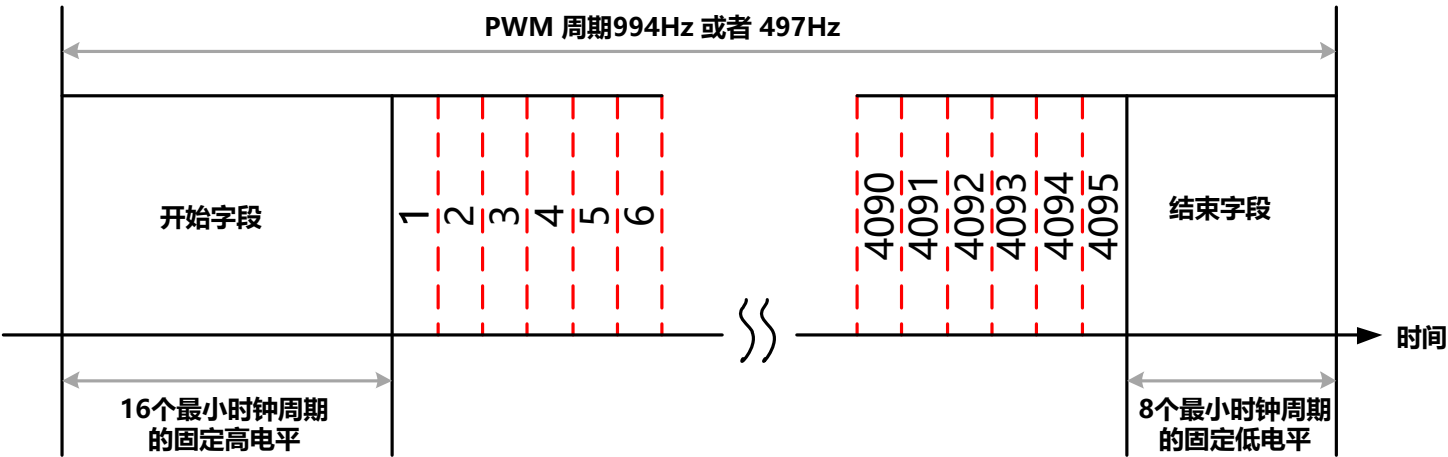
图-15: PWM输出
