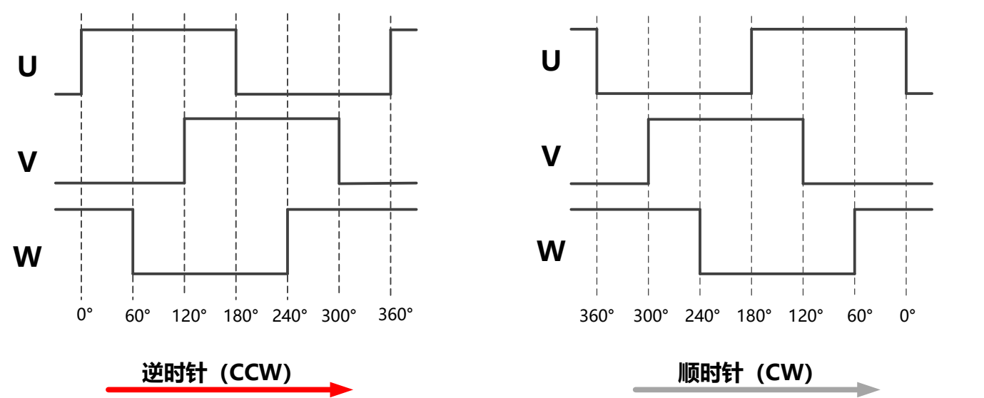
图-14: UVW输出波形
