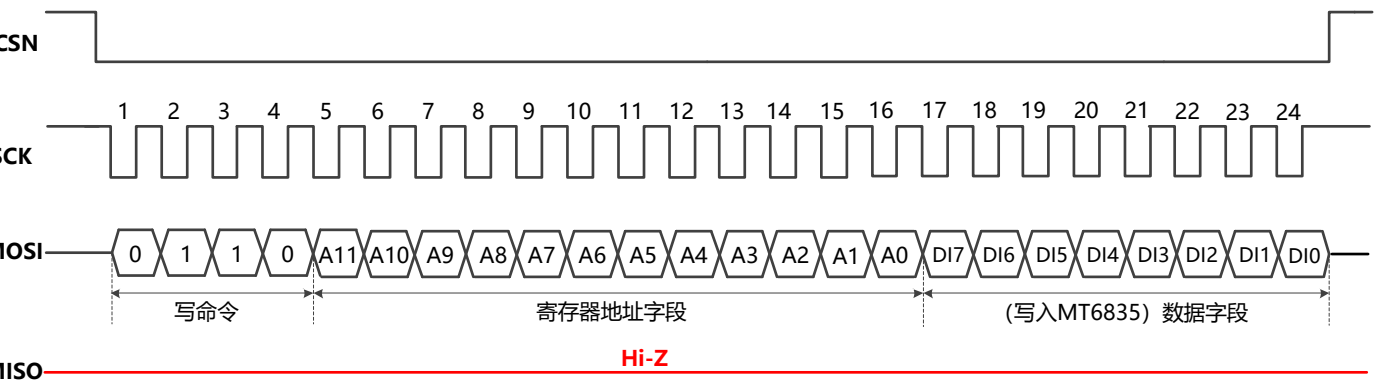
图-20: SPI单字节写寄存器
