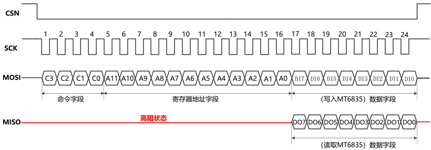
图-18: 4线SPI协议时序
