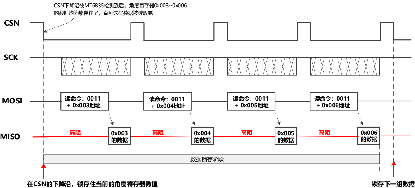
图-24: SPI 单字节读取角度寄存器
