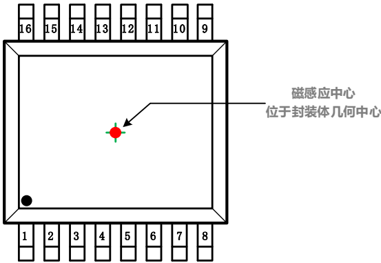
图-1: MT6835 TSSOP-16封装外观图
