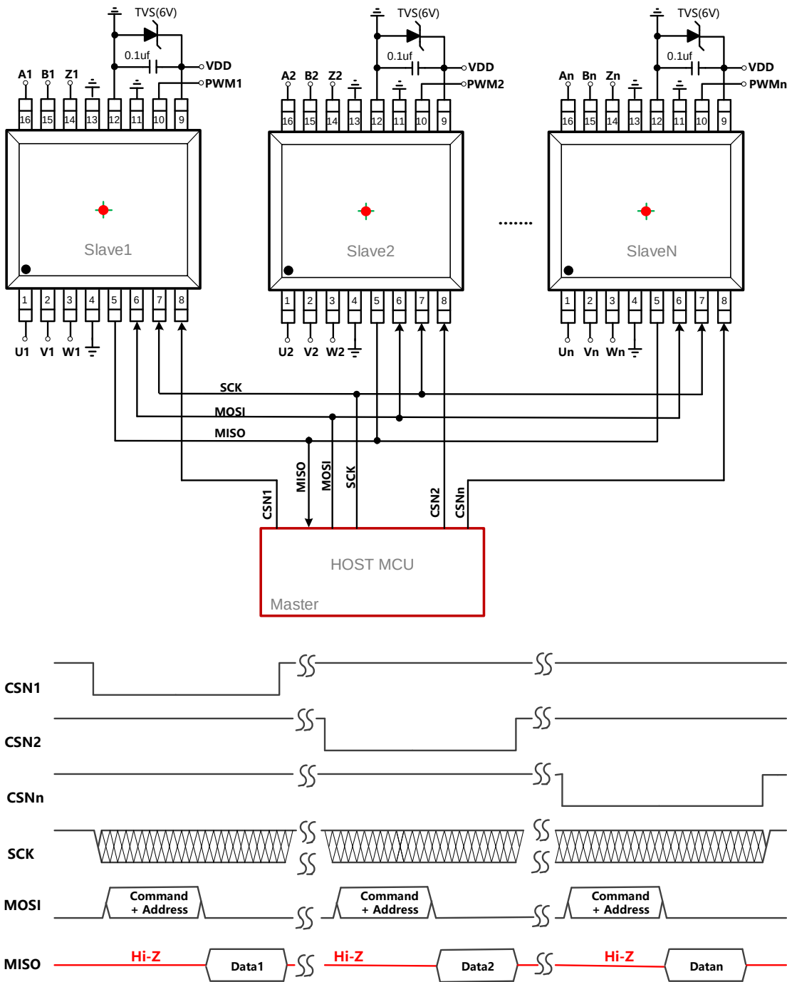
图-16: 4线SPI参考电路 (多芯片并联)
