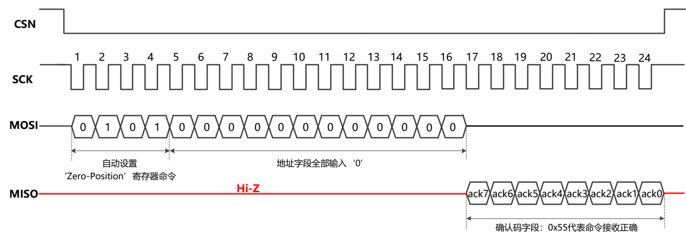
图-23: SPI 自动设置零点寄存器命令操作
