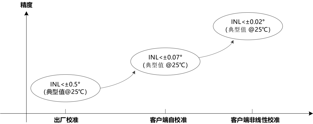
图-27: 三层校准
