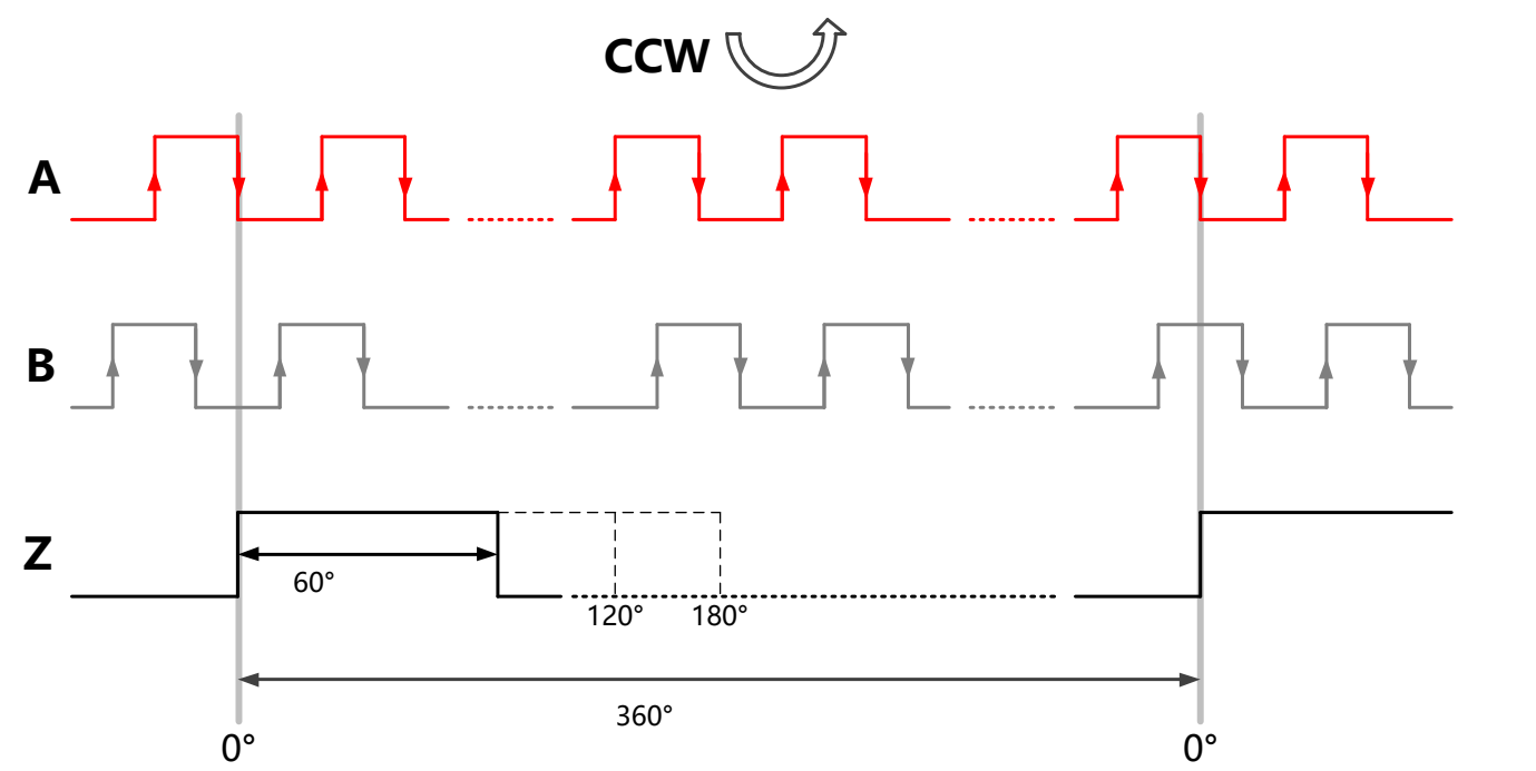
图-11: Z信号宽度=60°、120°、180°示意图
