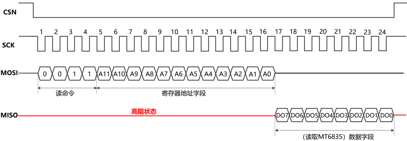
图-19: SPI单字节读寄存器
