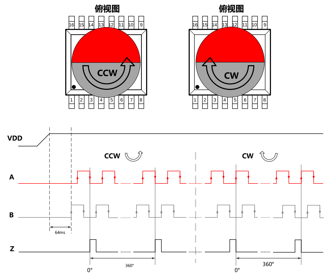
图-7: ABZ输出模式
