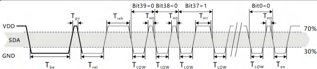
图9. AM2120单总线通信时序
