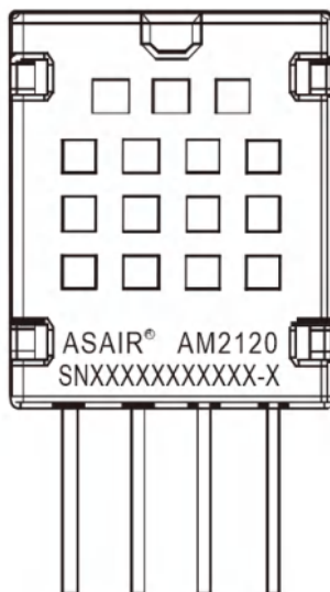
图 13. AM2120 传感器激光标识
