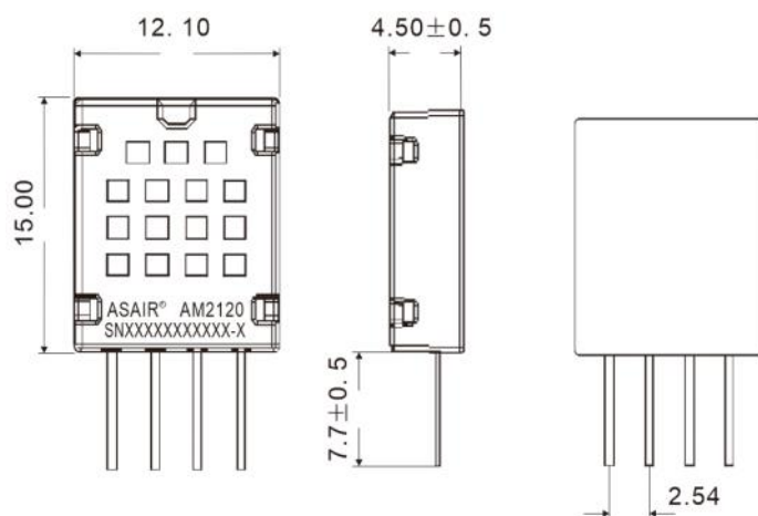
图5. AM2120尺寸图（单位：mm，其他公差：±0.1mm）
