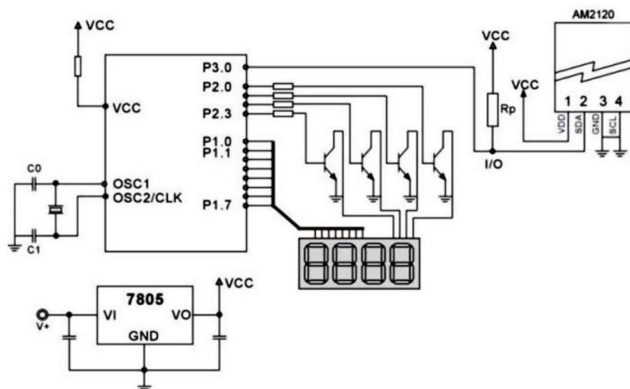
图6. AM2120单总线典型电路
