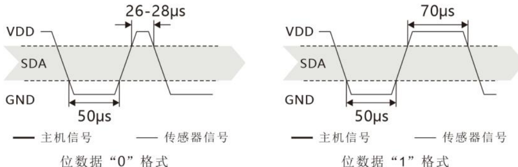
图12. AM2120发送数据位“0”和“1”示意图
