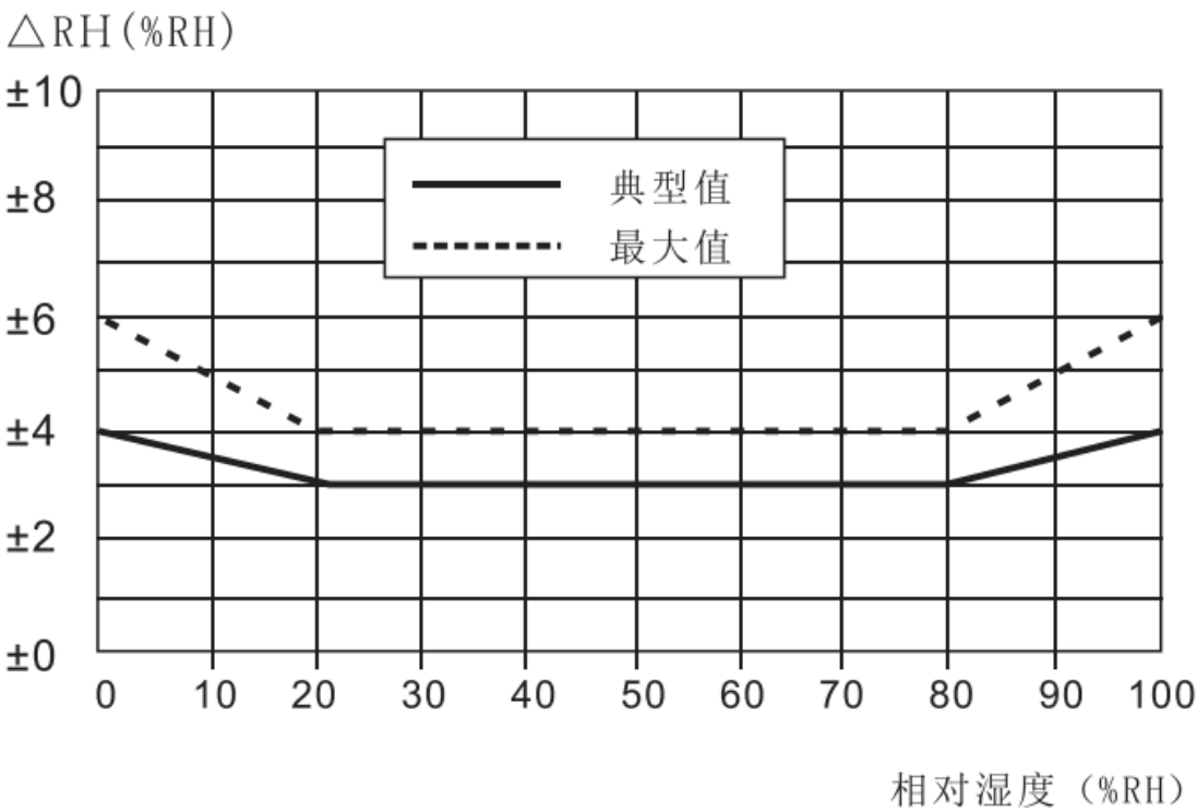
图 2. 25℃时相对湿度的最大误差
