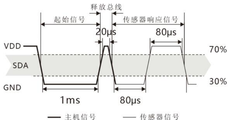
图11. 应答示意图
