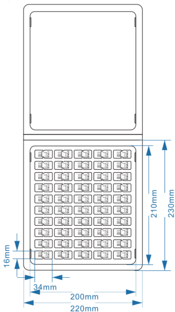
图 15: 吸塑盒和传感器定位图
