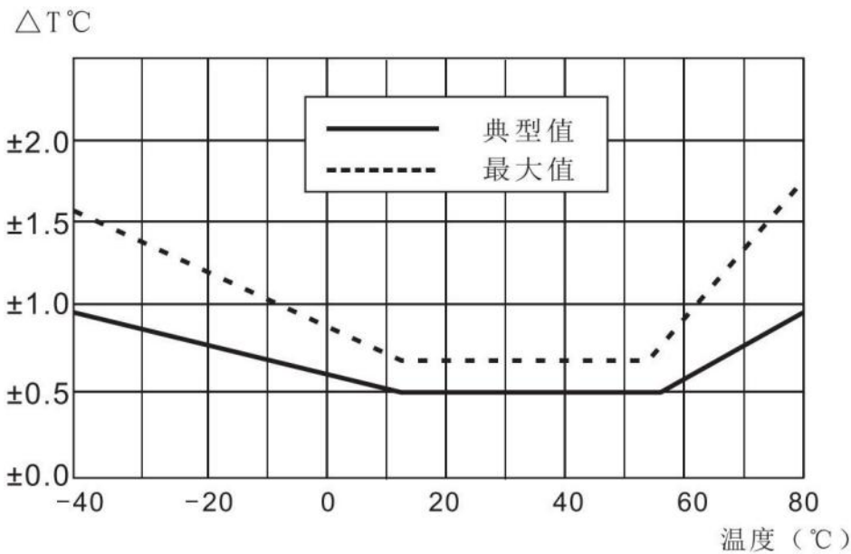
图 3. 温度典型误差和最大误差
