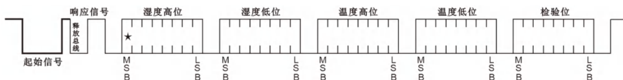
图7. AM2120单总线传送数据图
