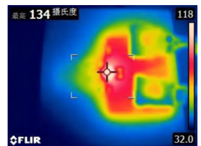
封装体热成像图（输入电流 45A）
