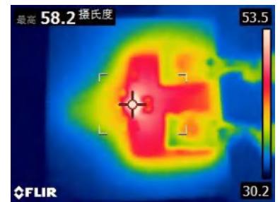
封装体热成像图（输入电流 25A）
