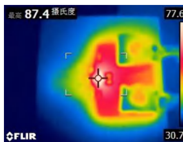
封装体热成像图（输入电流 35A）
