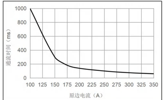
SOA 曲线
