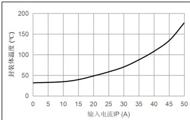
输入电流 IP vs. 封装温度
