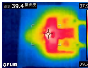
封装体热成像图（输入电流 15A）
