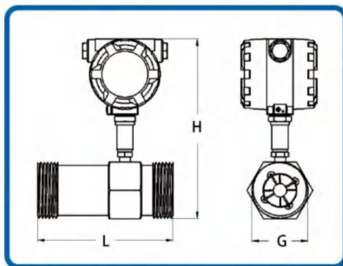
DN15 ~ DN50 螺纹连接传感器
