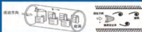
图2-1 涡街流量计工作原理示意图
