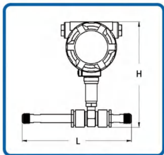
DN4 ~ DN10 螺纹连接传感器 (含直管段)
