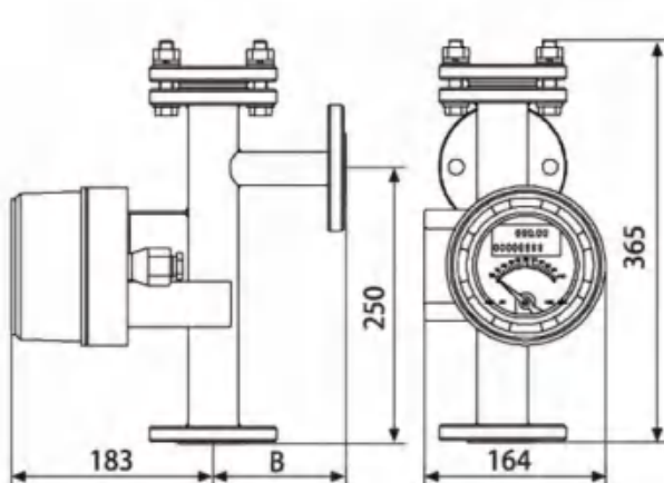
图4-12 标准型 M5 指示器
