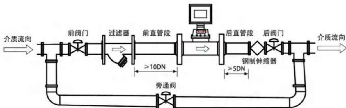
图8-1 典型安装管路系统
