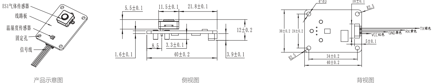
TB200B-ES1-Cl 2 -50-01尺寸示意图
