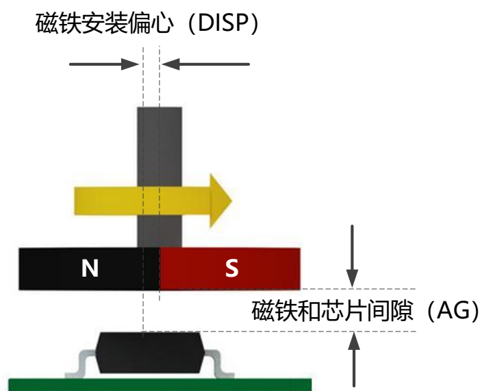
图-24: 磁铁安装
