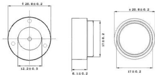
WK-21B超声波换能器
