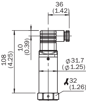
外壳尺寸图
