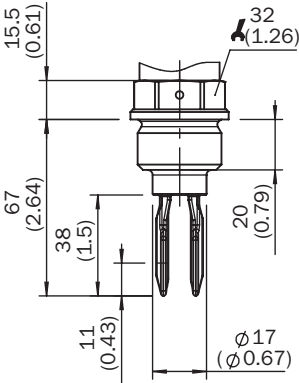
外壳尺寸图
