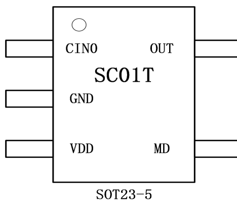
图1-1： 封装简图
