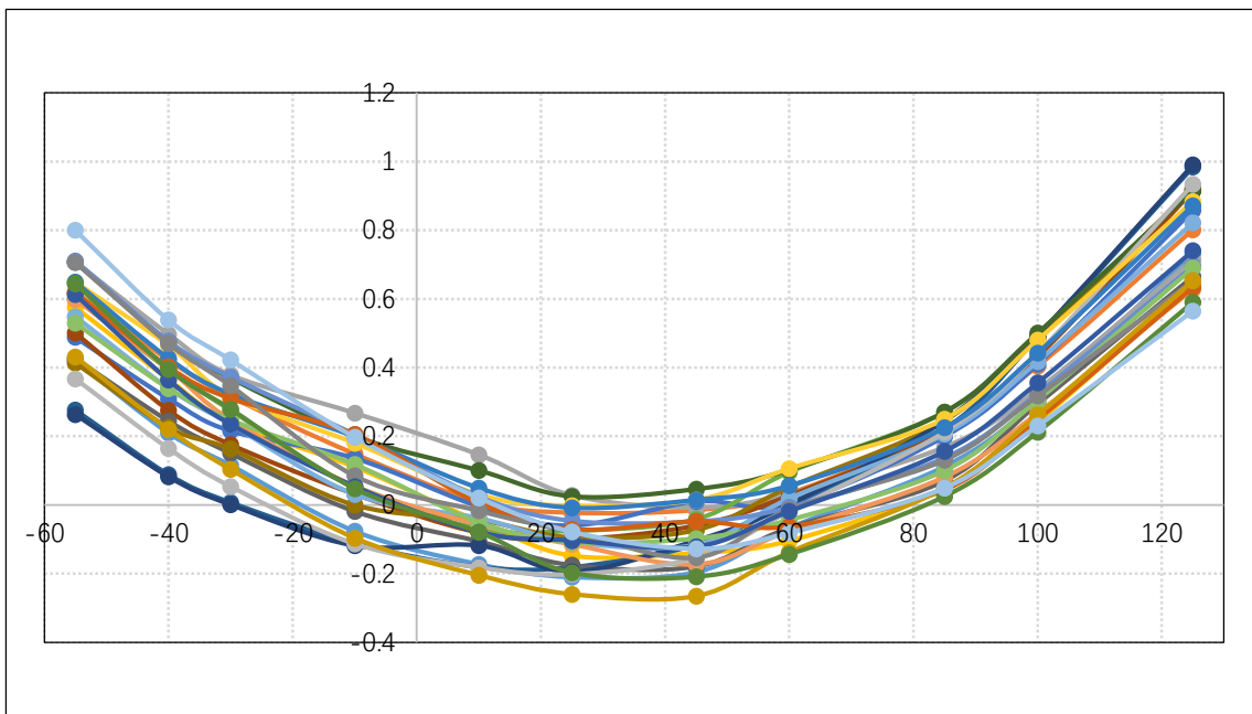
图 1-1 -55\sim 125^{\circ}\text{C} 典型温度误差曲线
