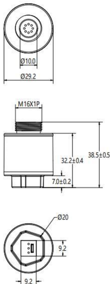
图2. AO-02外形尺寸图（单位：mm，其余未标注公差： \pm 0.2 mm）
