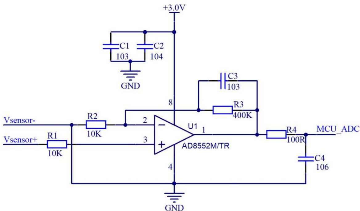
图 3. AO-02 推荐应用电路图
