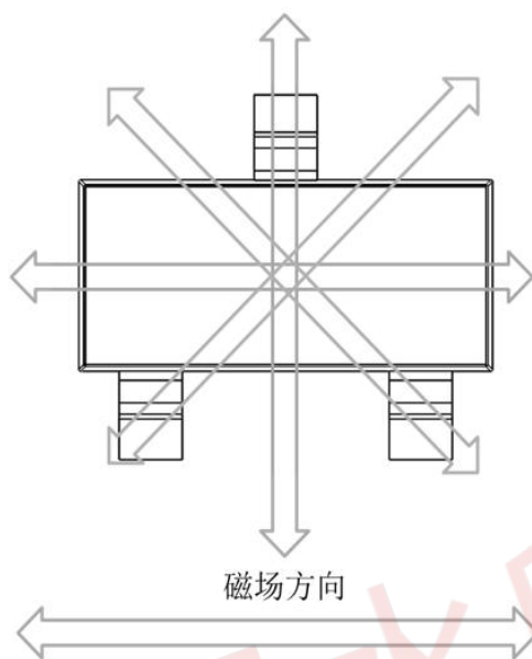
图3 SOT23-3L 封装感测方向图
