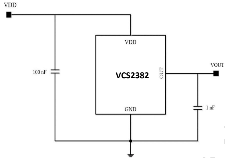
图 4 典型应用图
