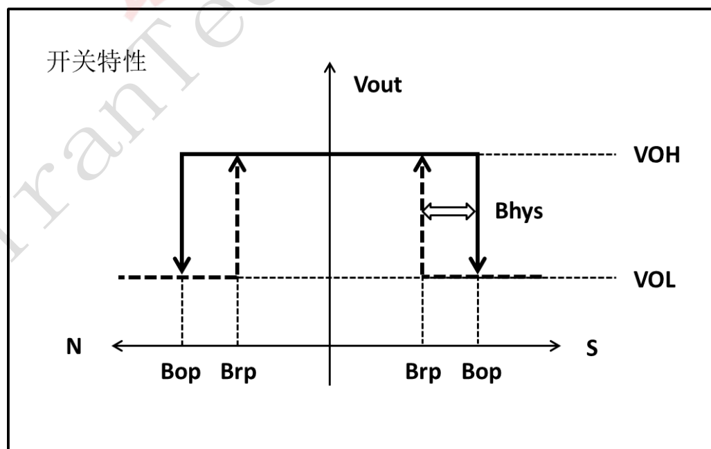
图4 开关特性图
