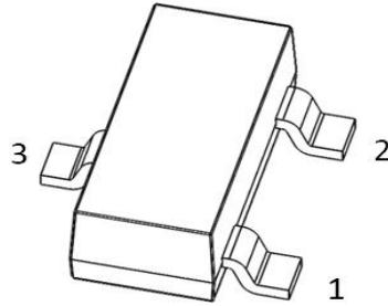
图 1 封装管脚示意图
