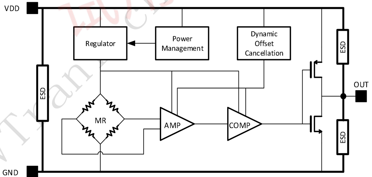
图 2 模块/线路图
